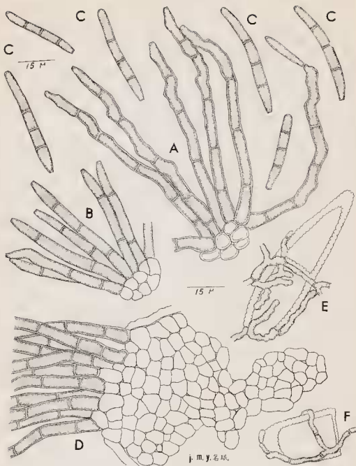
Fig. 1. Cercospora antholeiatae Yeu et Gilles (nov. sp.): A, Fascicule de conidiophores âgés; B, Fascicule de conidiophores jeunes; C, Conidies; D, Stroma et fascicule de conidiophores dense; E et F, Téléutospores du Puccintosira antholeiatae parasitées.
